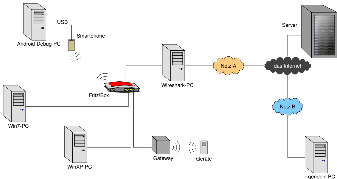
Abbildung 2: Schematischer Testaufbau
